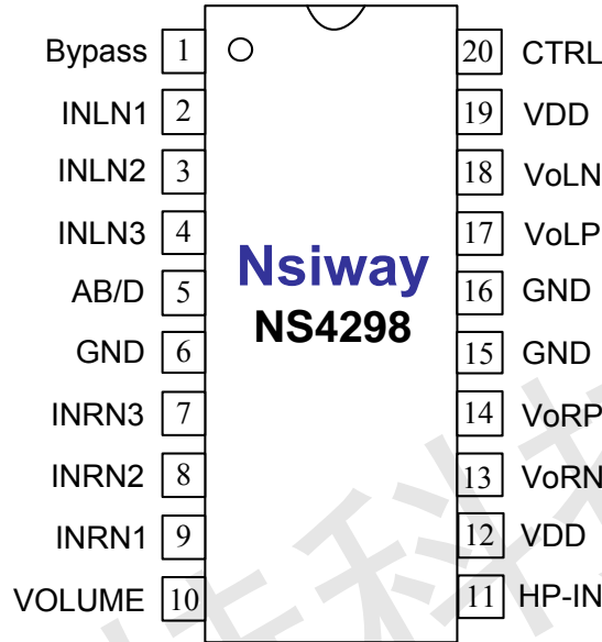
图2 TSSOP-20 管脚分配图(top view)
