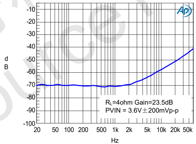
PSRR
