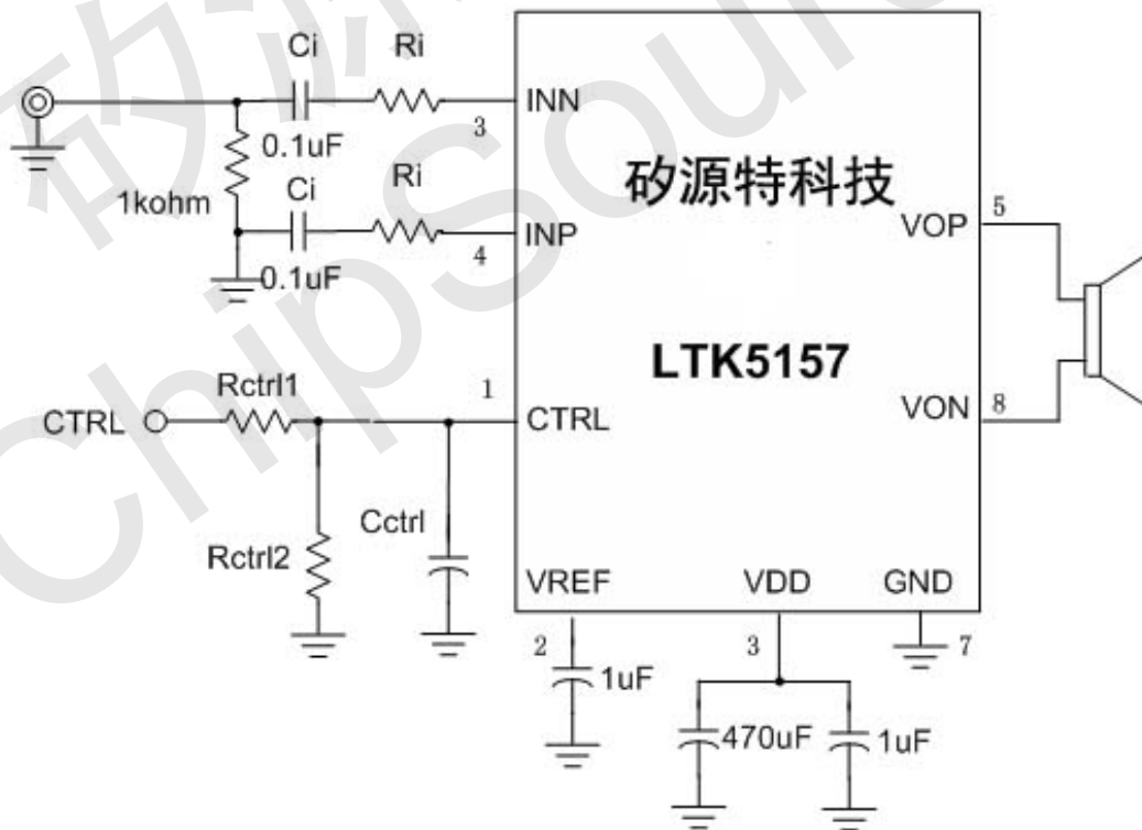
图五 LTK5157 单端输入带 ALC 防破音控制
