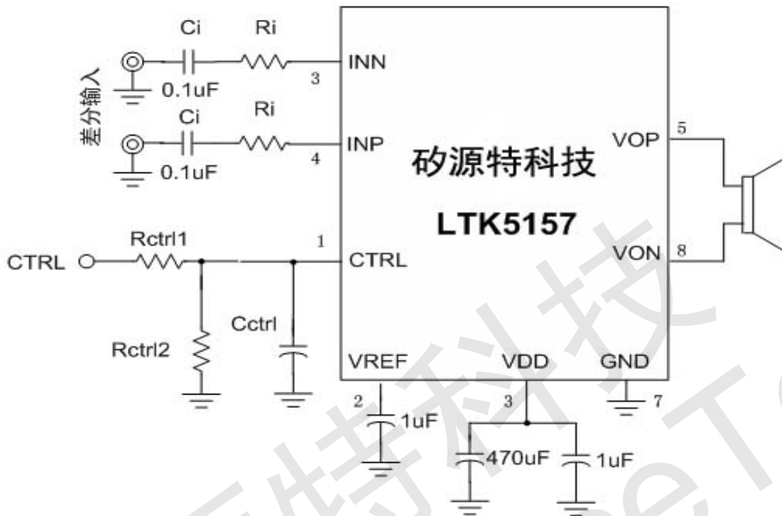
图四 LTK5157 差分输入带 ALC 防破音控制
