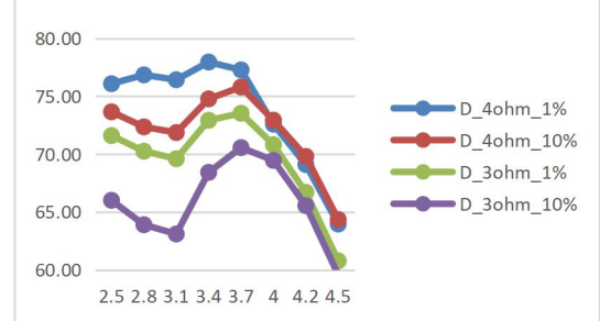
输出1W时D类 效率vs电源电压
