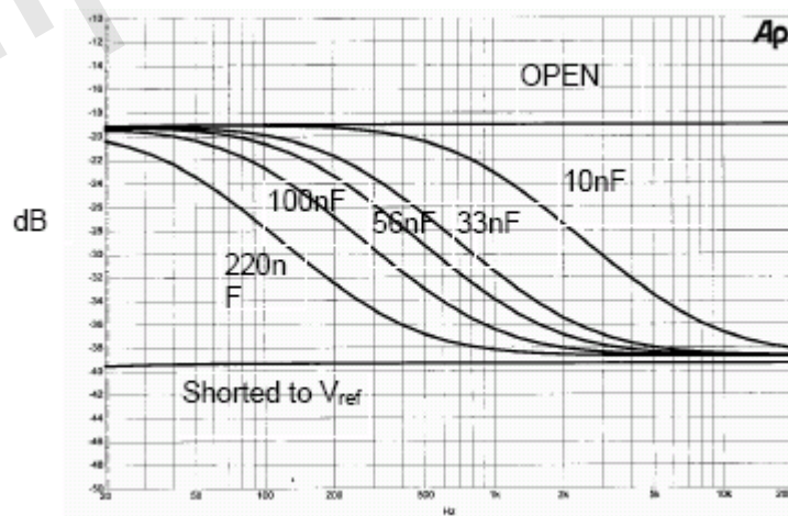
CST2314 C12、C13对响度的频率响应图 (Volume=-40Db, All other control flat)
