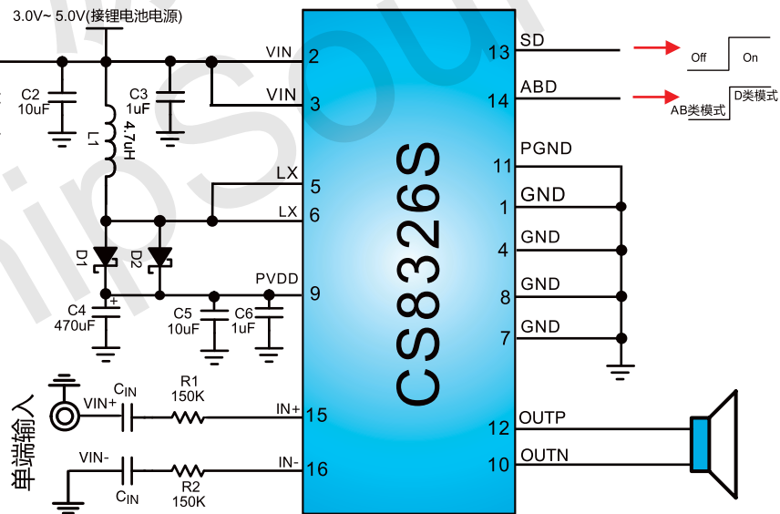
图 2 CS8326S单端输入方式应用图
