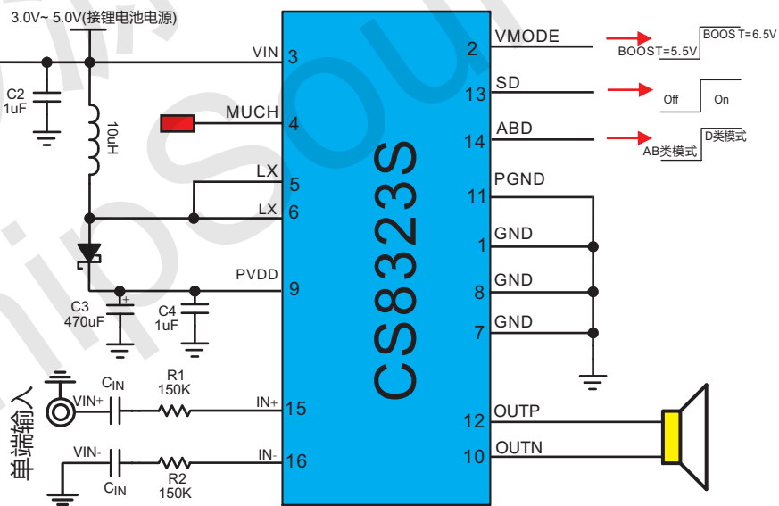
图 2 CS8323S单端输入方式应用图
