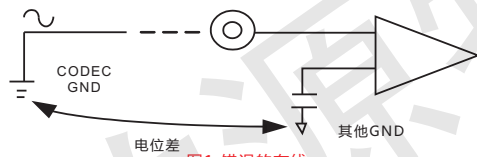
图1 错误的布线 ×
