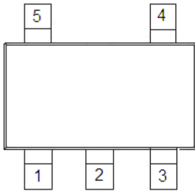
SOT23-5
