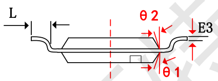
ESOP-8
