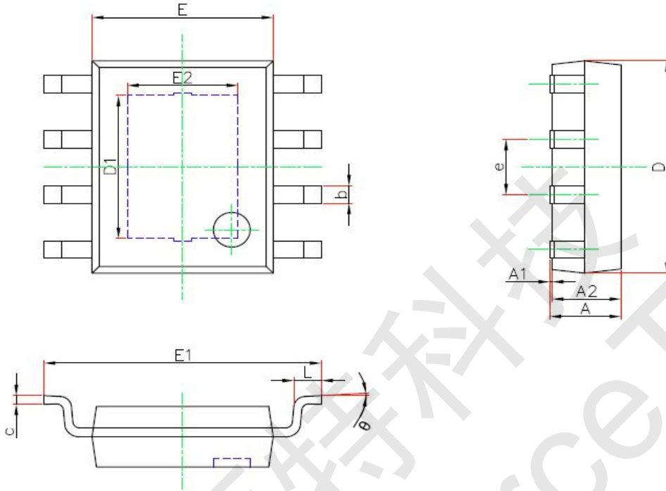
ESOP8 PACKAGE OUTLINE DIMENSIONS
